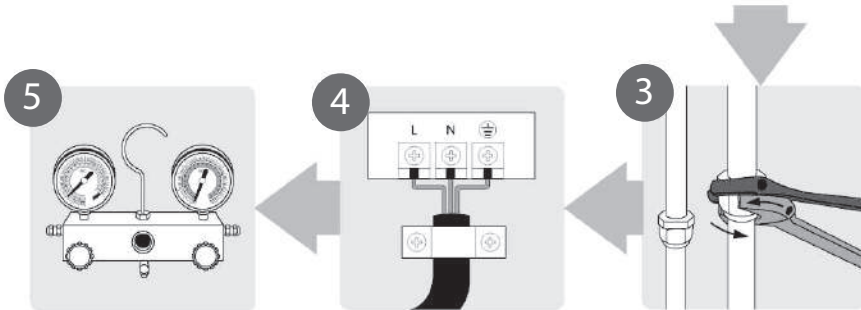
Сброс давления из системы с хладагентом
